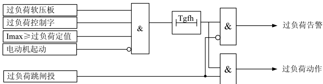
图 3-9 过负荷保护原理框图
