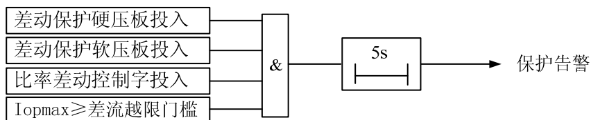
图 3-4 差流越限告警逻辑
