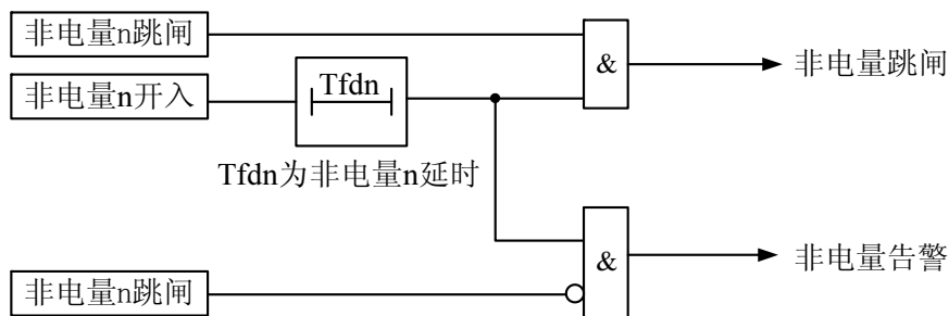
图 3-10 非电量保护逻辑
