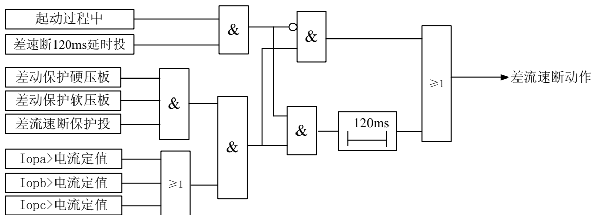
图 3-2 差流速断保护原理框图
