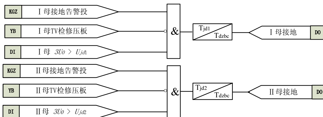
图 3-4 接地告警原理框图
