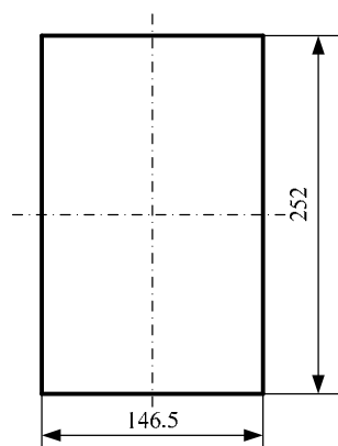
图 2-2 安装开孔尺寸
