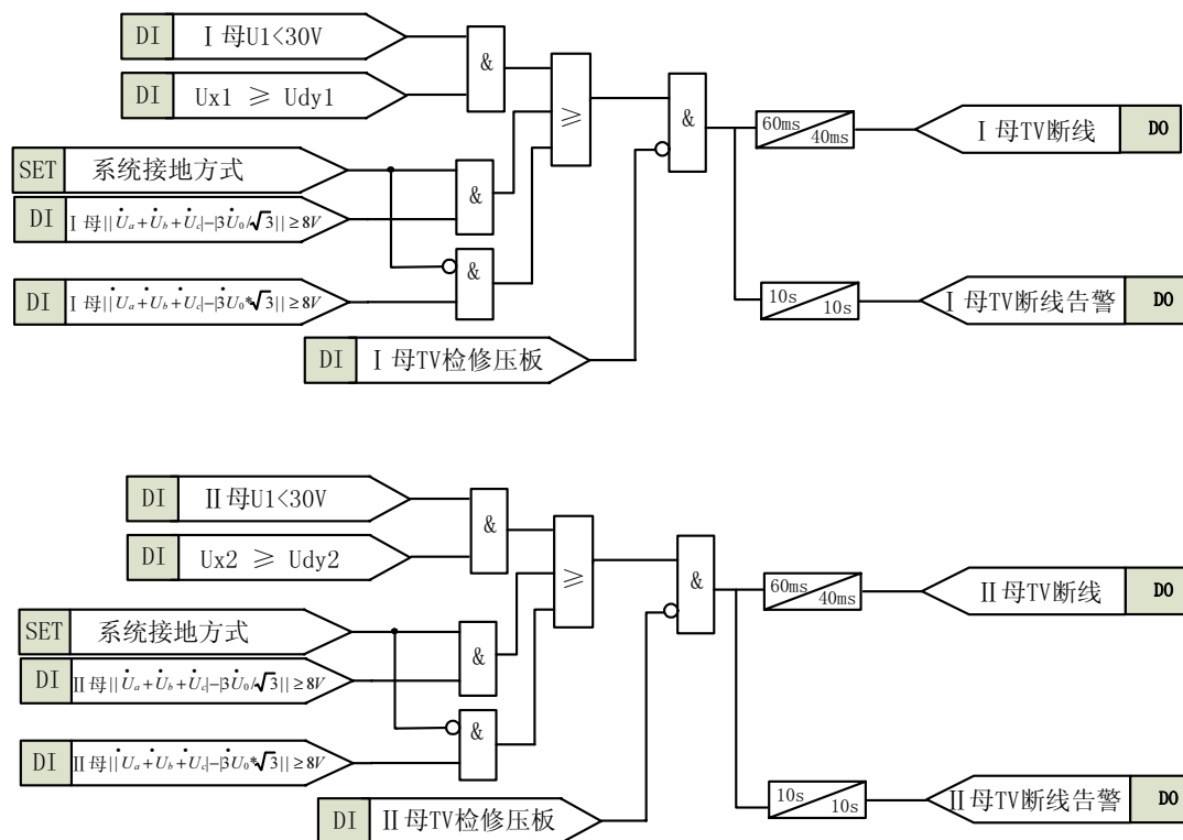
图 3-5 TV 断线检测原理框图
