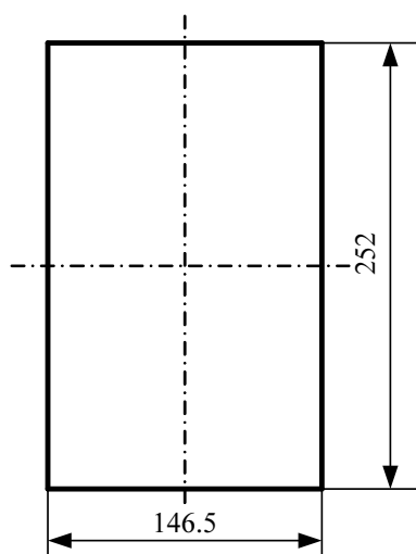
图 3-2 安装开孔尺寸
