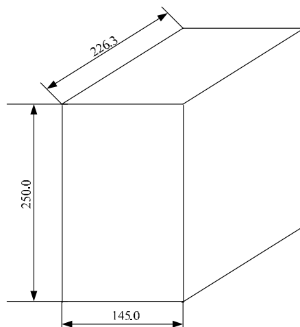
图 3-1 外形尺寸
