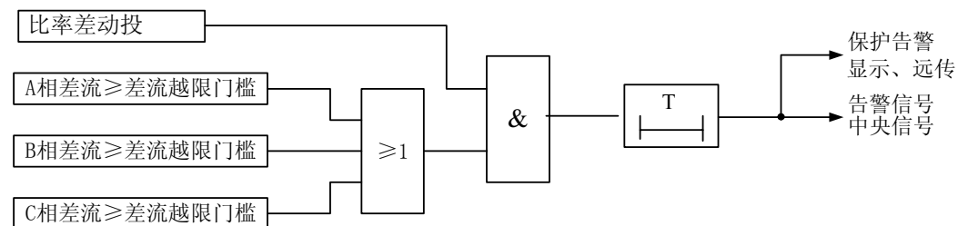
图 4-5 差流越限告警逻辑
