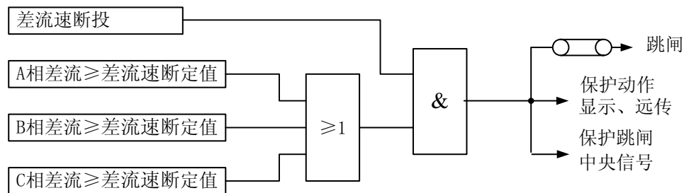
图 4-4 差流速断保护逻辑
