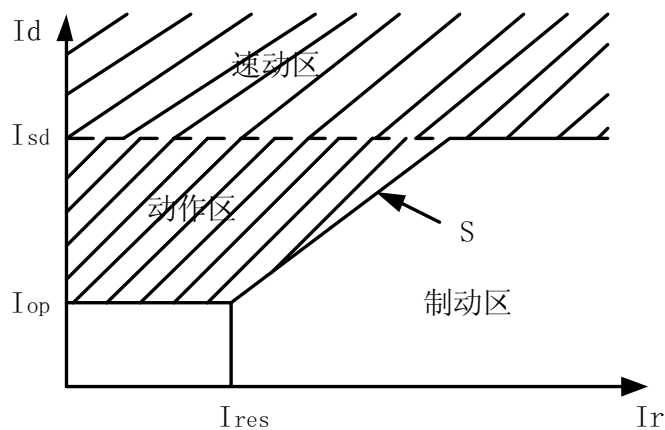
图 4-2 比率差动动作特性
