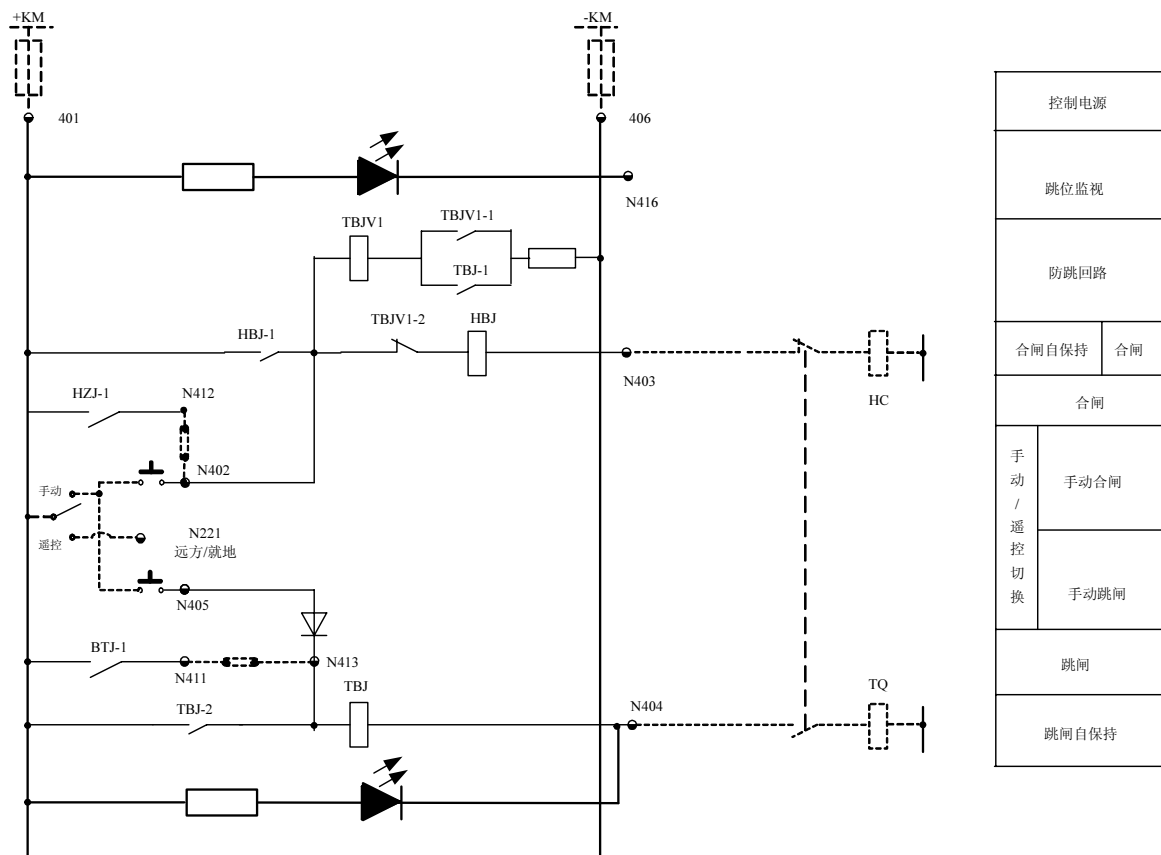
图 12-2: 装置操作回路原理图
