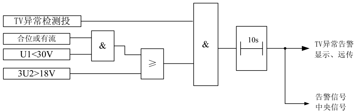
断线告警原理框图
