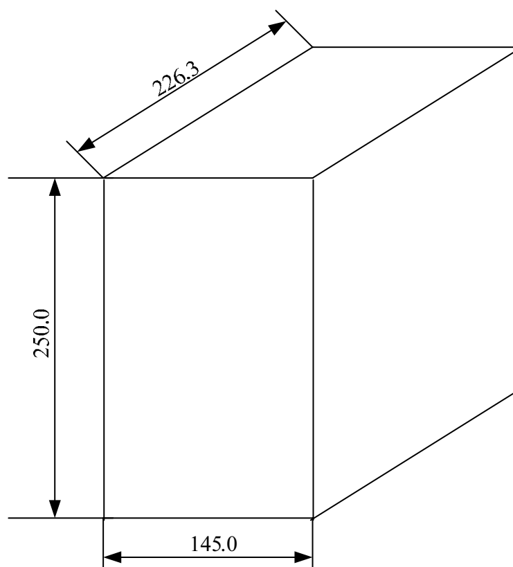
图 3-1 外形尺寸
