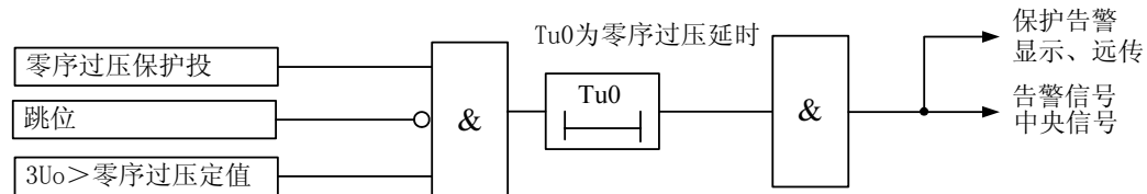
图 4-10 零序过压保护逻辑
