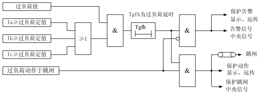
图 4-9 过负荷保护原理框图
