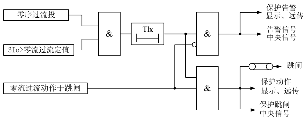
图 4-8 零序电流保护原理框图
