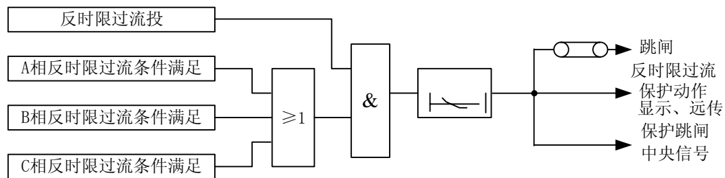
图 4-7 反时限过流保护逻辑
