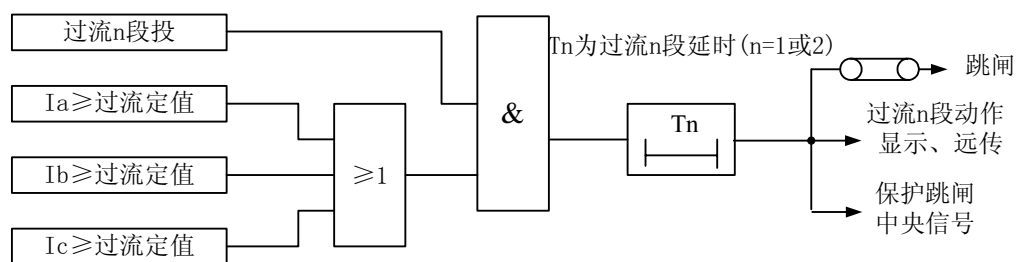
图 4-6 过流保护逻辑
