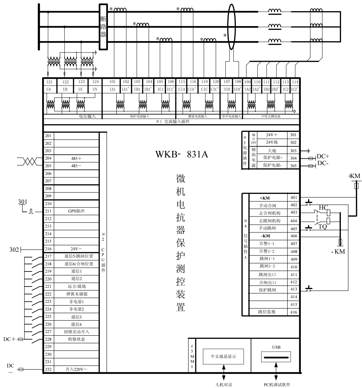
图 12-1: WKB-831A 装置接线示意图
