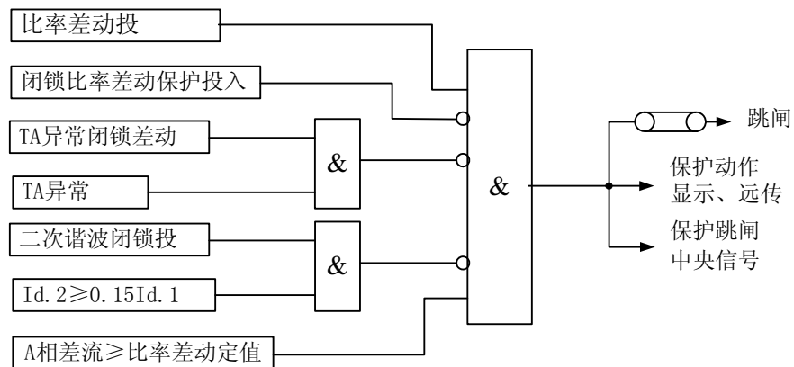
图 4-3 比率差动动作逻辑图
