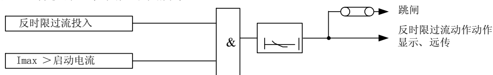
图 3-2 反时限过流保护原理框图
