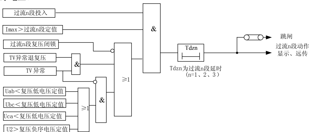
图 3-1 复压闭锁过流保护原理框图
