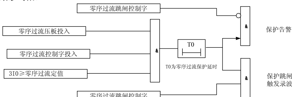
图 3-4 高压侧零序过流保护原理框图
