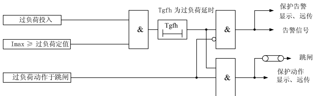
图 3-3 过负荷保护原理框图
