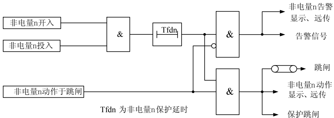
图 3-7 非电量保护原理框图
