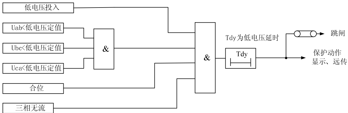
图 3-5 低电压保护原理框图
