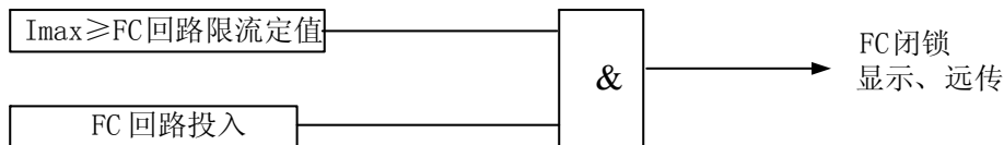
图 3-8 FC 回路保护原理框图
