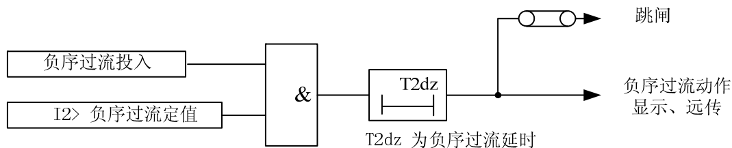
图 3-6 负序过流保护原理框图
